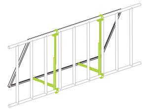
Système de montage pour balcon
