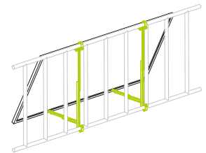
Система крепления для балкона
